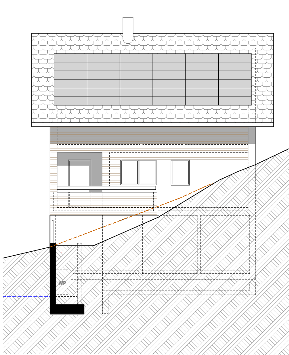
ANSICHT SÜDEN Haus D
