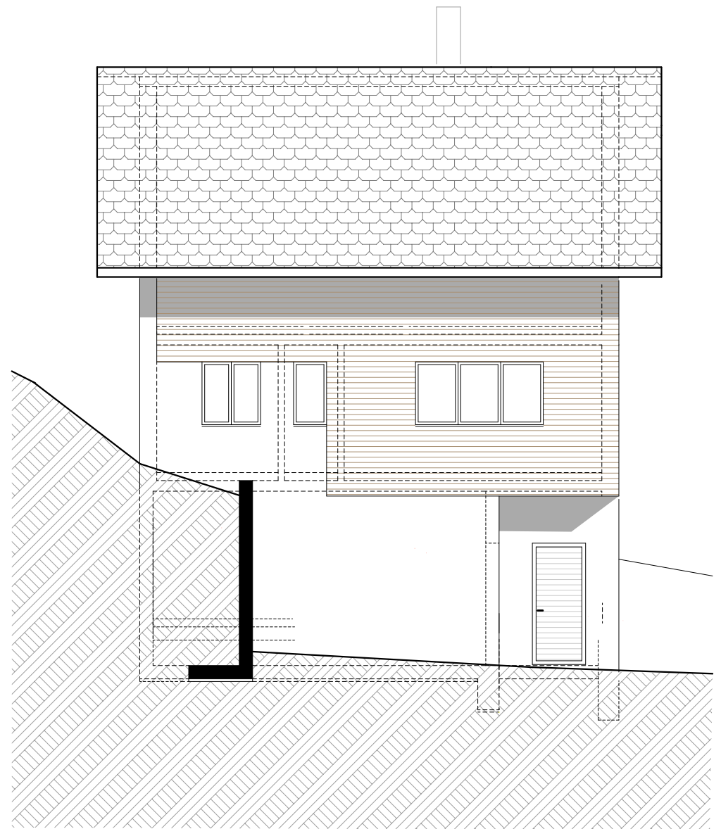
ANSICHT NORDEN Haus D
